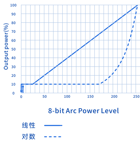
调光曲线
